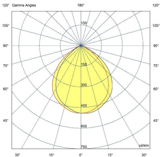
СВЕТЛОРАЗПРЕДЕЛИТЕЛНА ДИАГРАМА
