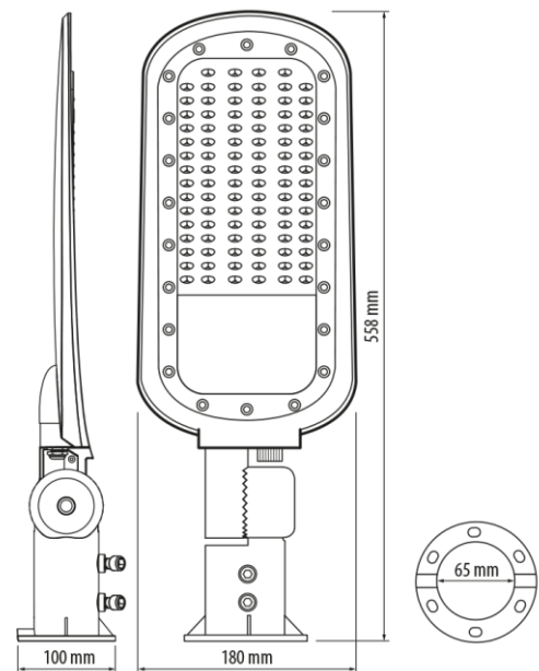
РАЗМЕРИ
